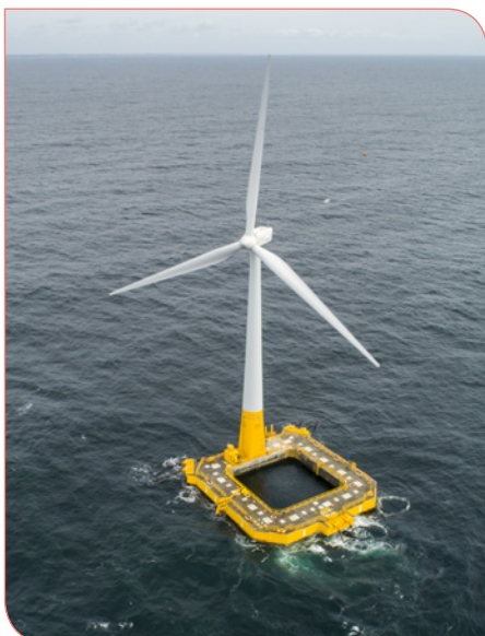
Floatgen ©Ideol BYTP ECN V. Joncheray
